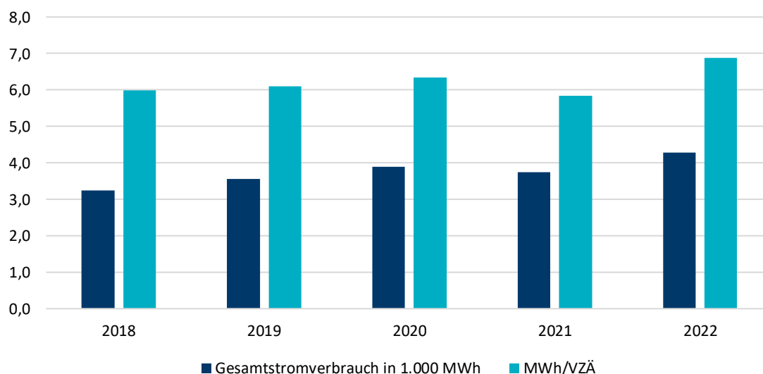
Abbildung 7: Gesamtstromverbrauch in 1,000 MWh bzw. MWh/VZÄ von 2018 bis 2022
